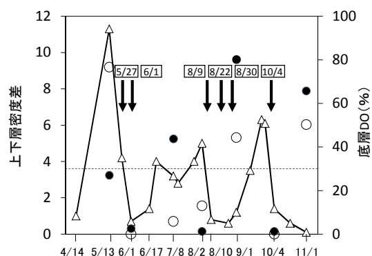
図3 2016年の航路・泊地沖の上下層密度差(Δ: St. 2)及び航路・泊地の底層DO(●: St. 1, ○: St. 3)の推移 矢印は苦潮発生日を、破線は貧酸素水塊の基準とした底層DO30%を示す。
