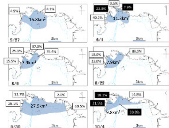
図2 2016年の蒲郡市地先の航路・泊地から発生した苦潮の範囲及び表層DO(%) (黒字: 陸上観測, 白字: 海上観測)
