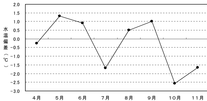
図4 伊勢湾（三河湾）表面水温の平年偏差
