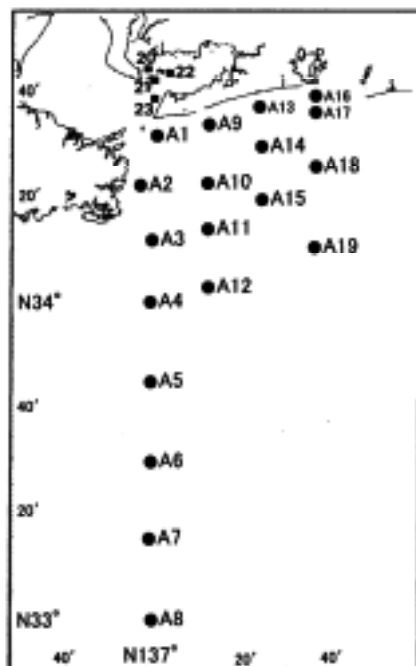
図1 沿岸定線観測定点 (A5～8については4，2，3月のみ実施)
